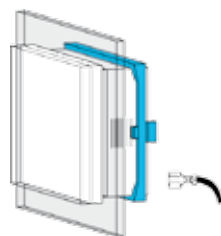
Inbouwmontage; aansluiting via fast-on stekkers 4,8 mm
