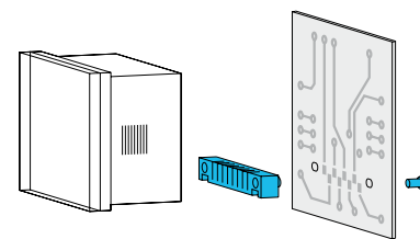
Montage op printplaat met aansluitstrook, ref. 907 5 141
